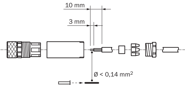
Монтажный чертеж
