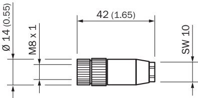
Габаритный чертеж (Размеры, мм)
