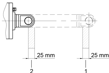
Abb. 4 Reducción máxima de la carrera
