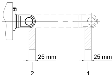
Abb. 4 Réduction maximale de la course
