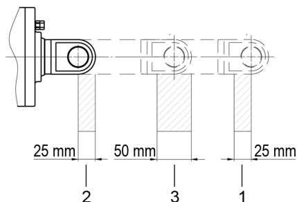
Abb. 7 Campo di regolazione ammesso della posizione intermedia
