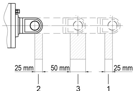
Abb. 7 zulässiger Verstellbereich Zwischenposition
