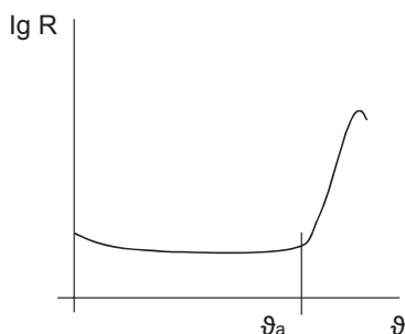
Abb. 3 Courbe caractéristique R- \theta d'un élément chauffant CPT
