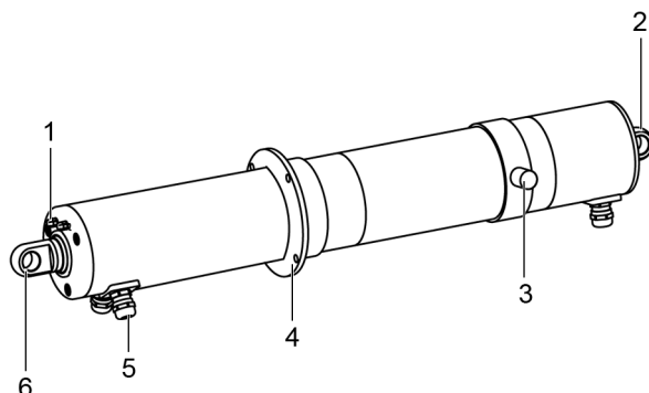
Abb. 1 Composants d'un vérin
