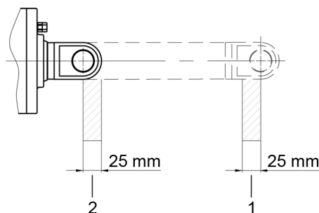
Abb. 4 massima riduzione della corsa
