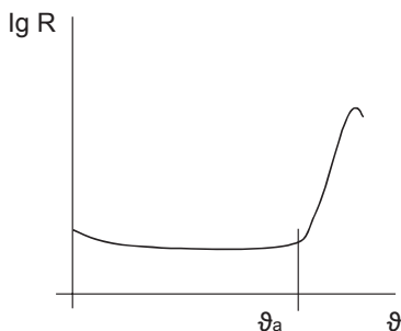
Abb. 3 R- \theta -Kennlinie eines PTC-Heizelements
