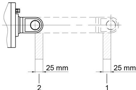
Abb. 4 maximale Hubminderung
